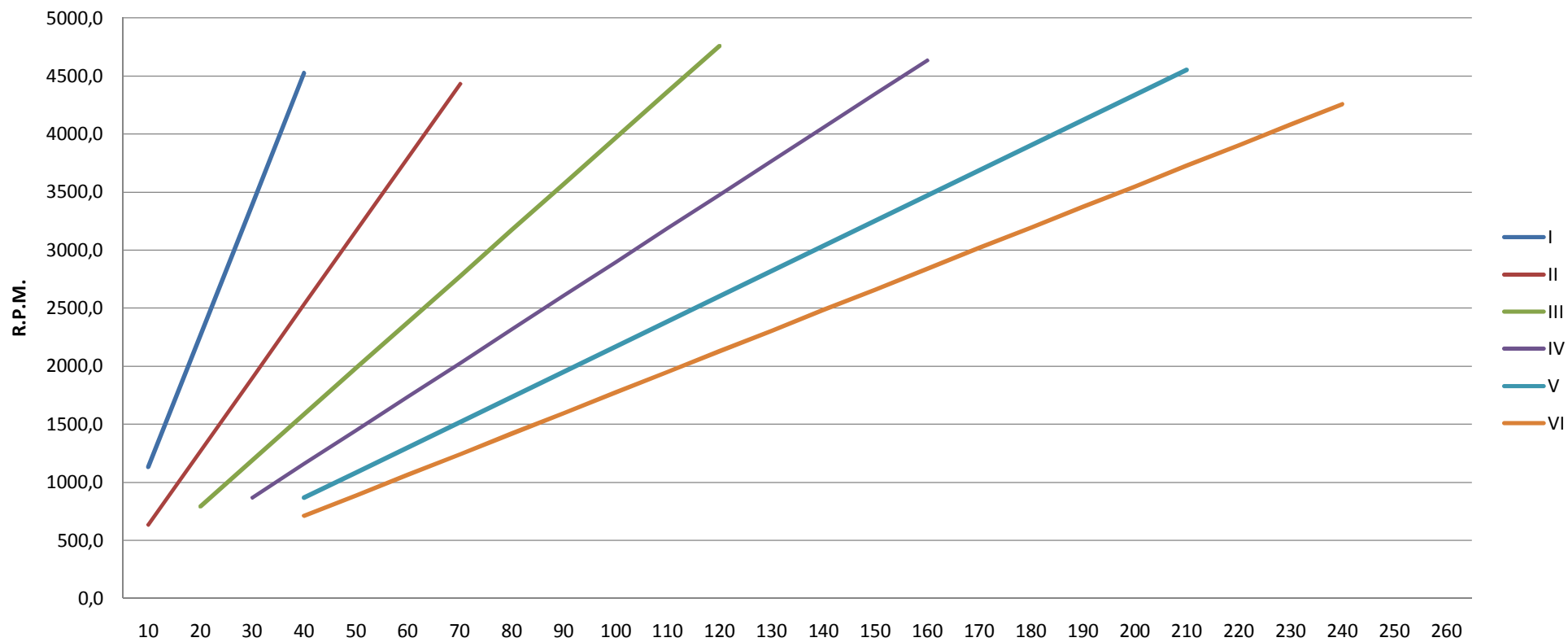
Velocidad para cada marcha en funcion rpm
